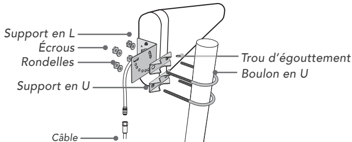
Montage de l'antenne Yagi
