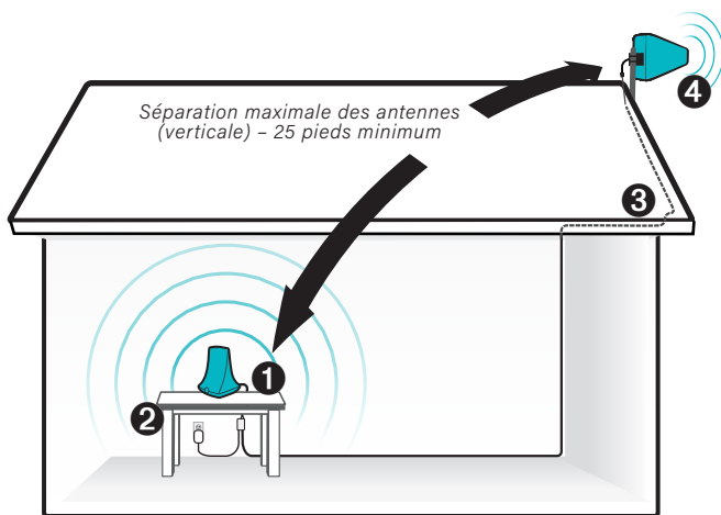
Aperçu de l'installation
